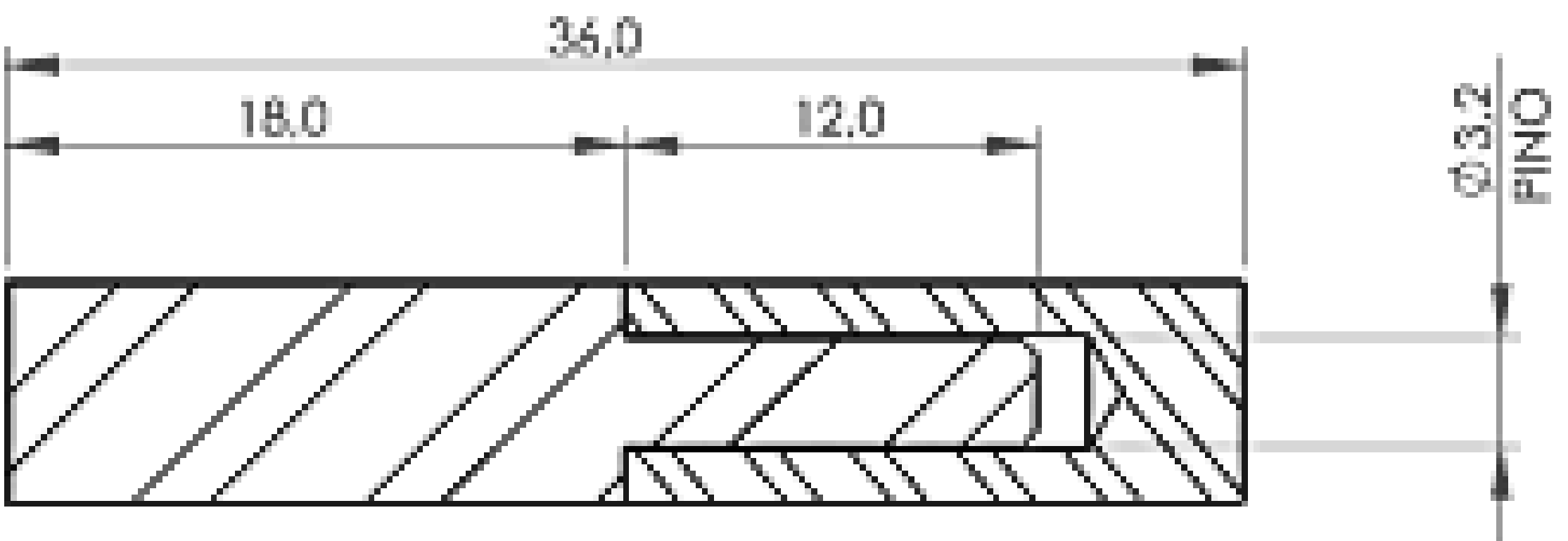
SEÇÃO A-A
