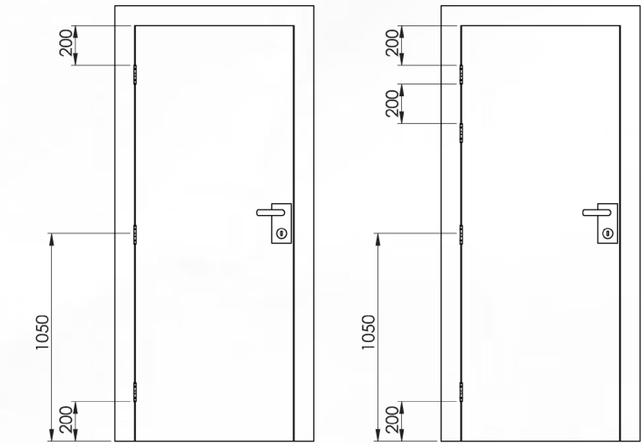
3 DOBRADIÇAS
